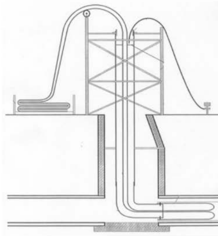
Abbildung 1: Darstellung Inversionsvorgang, in Anlehnung Deutsches Institut für Bautechnik (DIBt)
